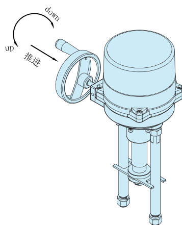
手动操作
